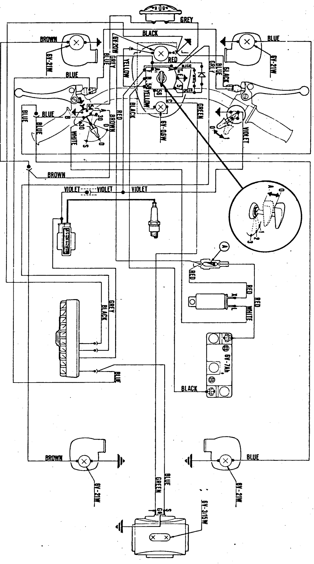
Fig. 1 - Wiring diagram
